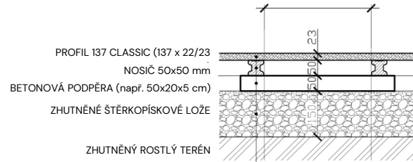
Obr. 1 Skladba terasy při použití nosičů Terafest® 50x50 mm
