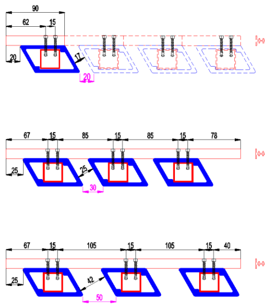
Vrutované spoje
