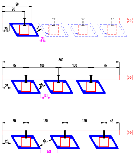
Nýtované spoje
