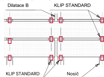
Obr. 5 Napojování terasových prken pomocí KLIPU STANDARD
